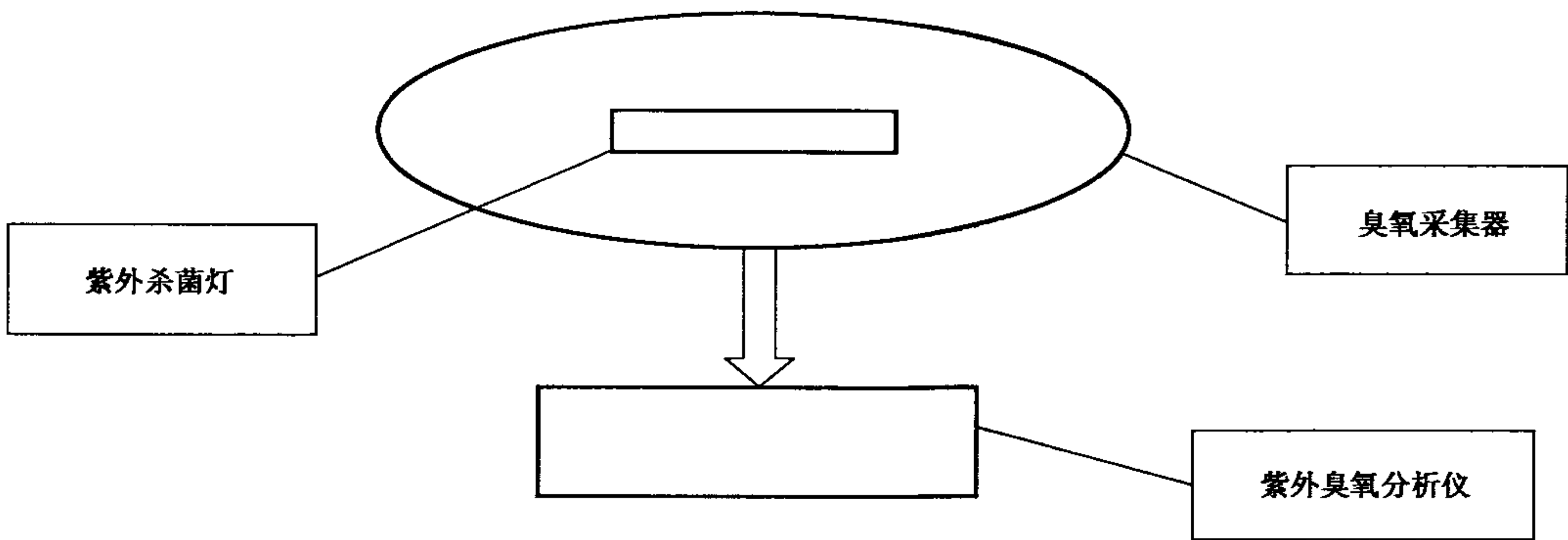
图 D.1 臭氧产出率测试系统
